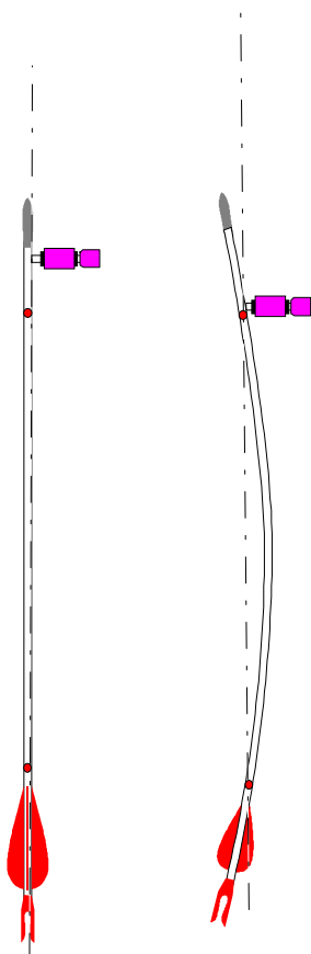
Figure 3: La flèche vibre pendant son vol autour de deux points relativement fixes: les noeuds de vibration.
