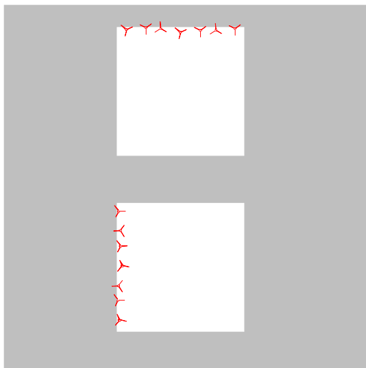
Figure 14: Réglage fin à courte distance
